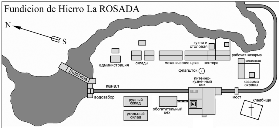
План металлургического завода «Ла Росада» в Ибикуи
